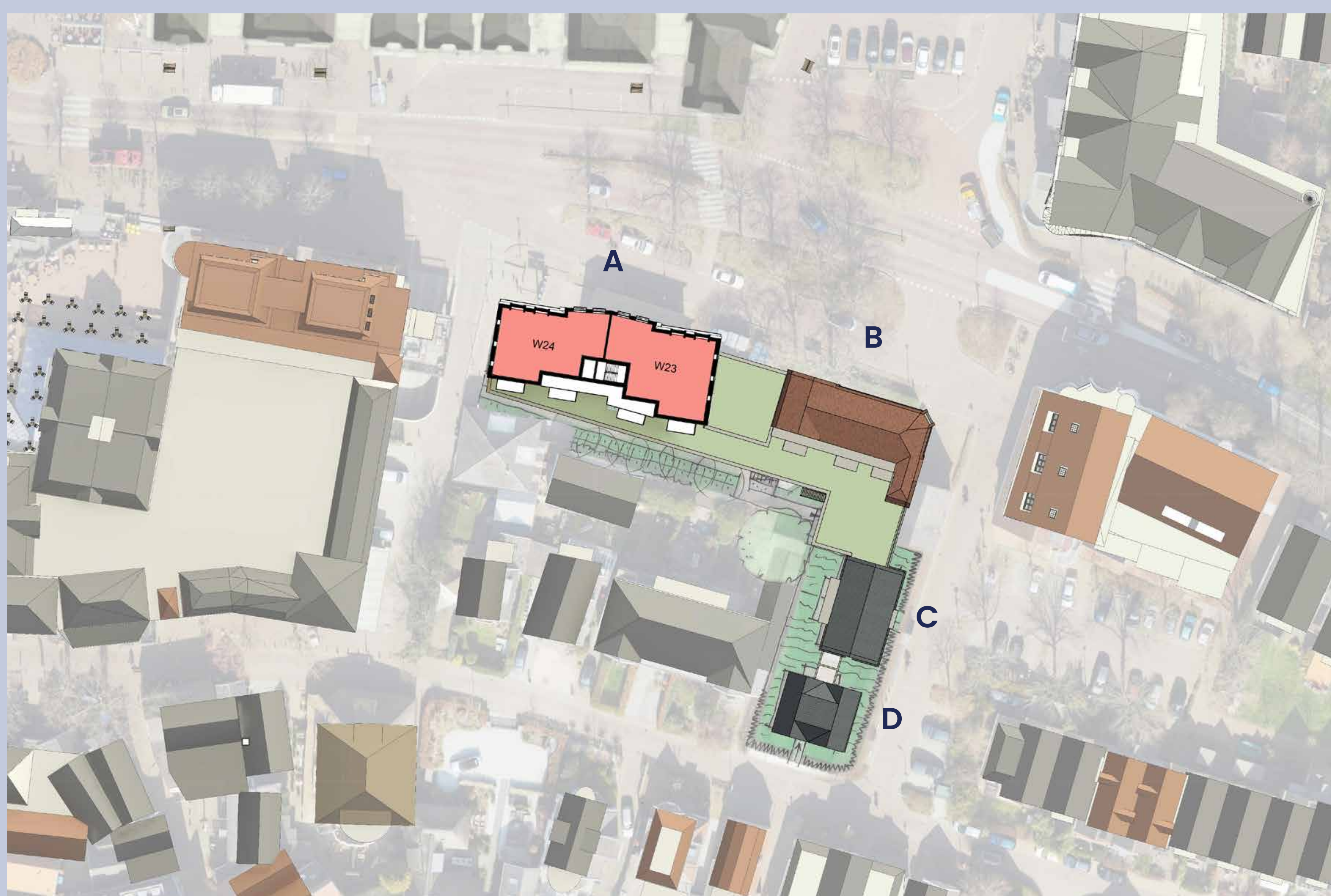
Plattegrond derde verdieping
